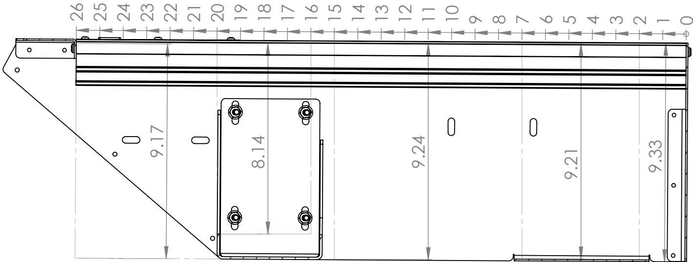
DS 9" WIDE SECTION
