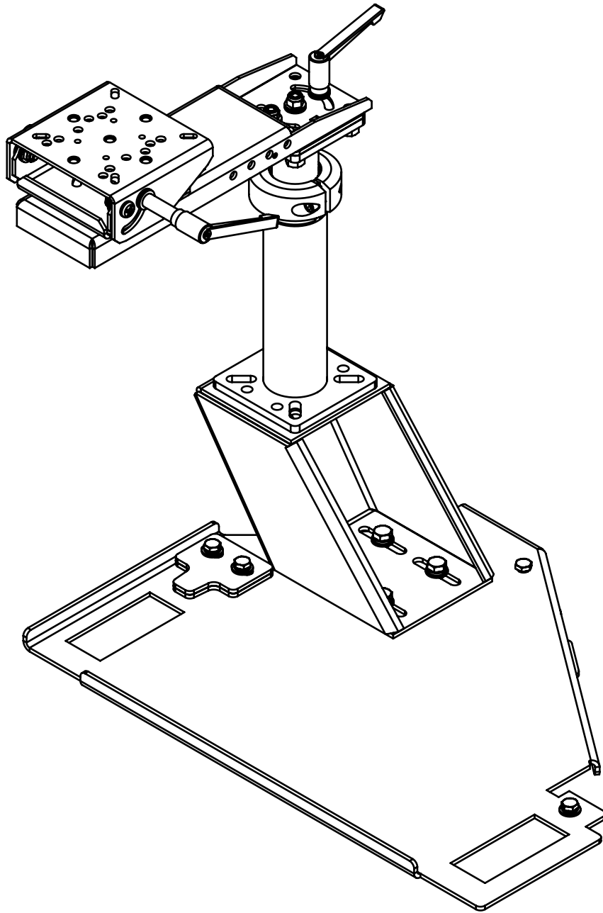
PKG-PSM-176
